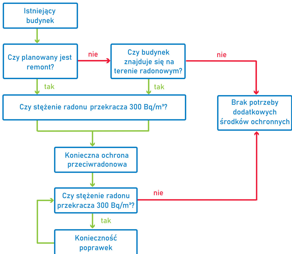
Rys. 3 Schemat procedury oceny i planowania działań ochronnych w istniejących budynkach w przypadku podwyższonego poziomu radonu 26
